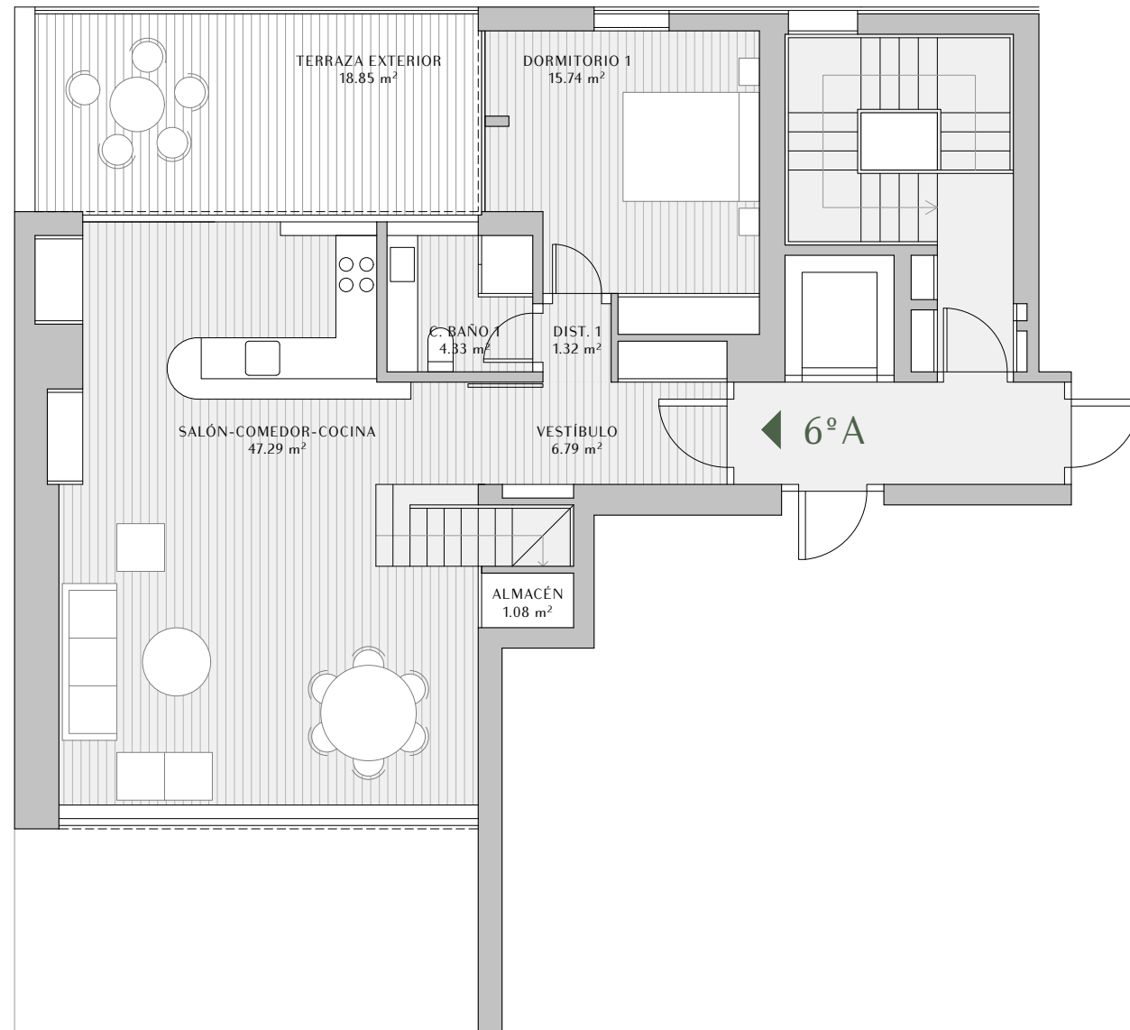
PLANTA BAJA
