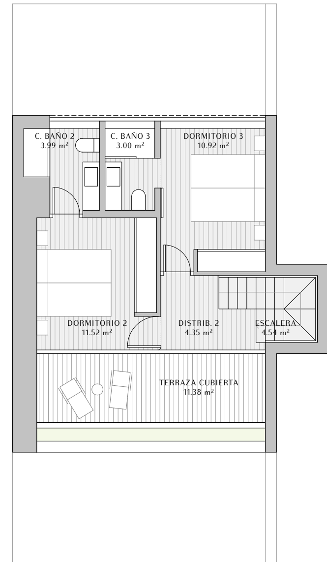
PLANTA PRIMERA
